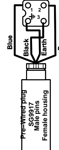
Detachable Motor Tail 0562
